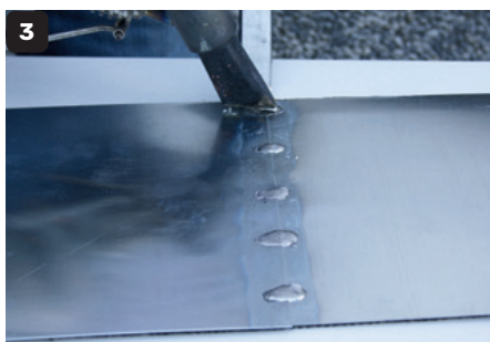
Vertinnen van de soldeerbout op de ammoniaksteen. Puntsoldering van de te solderen delen.
