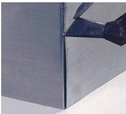
Puntsoldering
