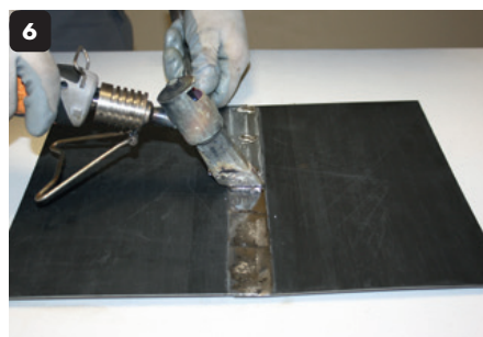
Breng Zinn 7 aan over de lengte van de soldeernaad. Soldering van de bladen (versterkte soldering).
