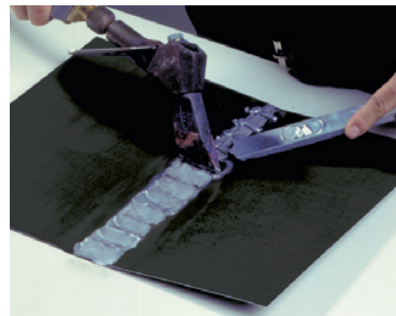
Traceren van de overlappende delen
