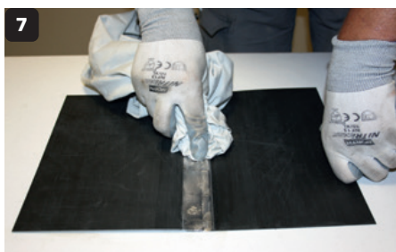
Afvegen met een zuivere doek.
