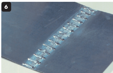
Reinig de soldeernaad met een zuivere vochtige doek met zuiver water.
